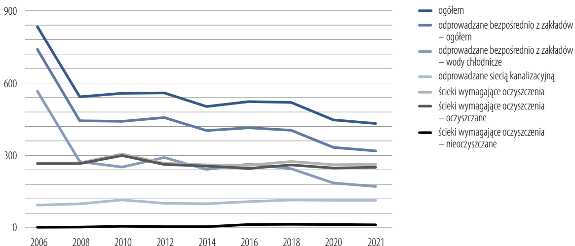
Wykres 2. Ścieki przemysłowe i komunalne odprowadzone do wód powierzchniowych lub ziemi w województwie małopolskim (w hm 3 /rok)
