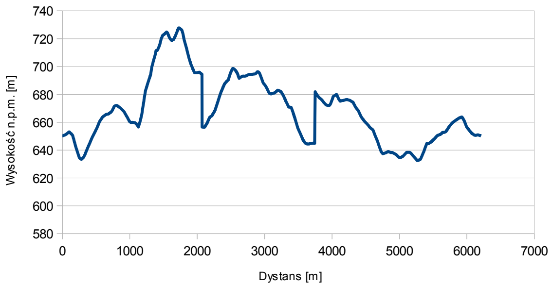
Rysunek 37: Przekrój podłużny trasy w Kluszkowcach.
